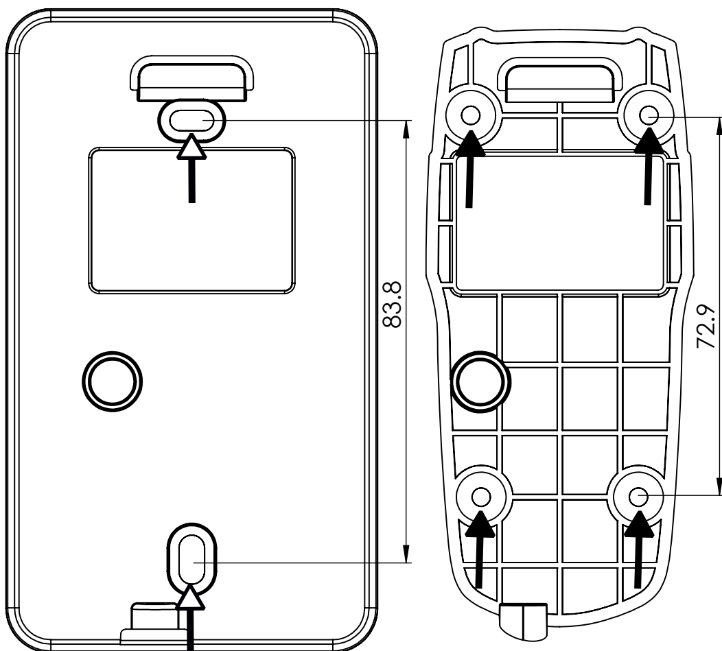
Furos para suporte de caixa 4x2
